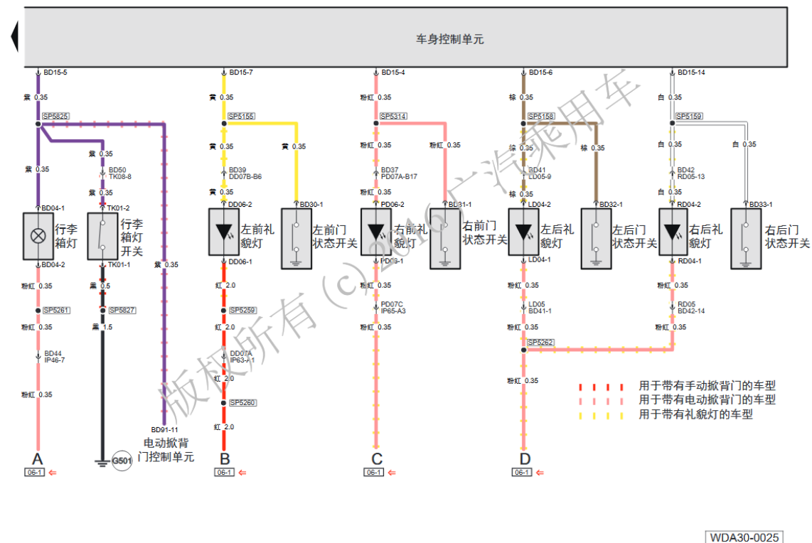
06-3 车内灯系统电路图
